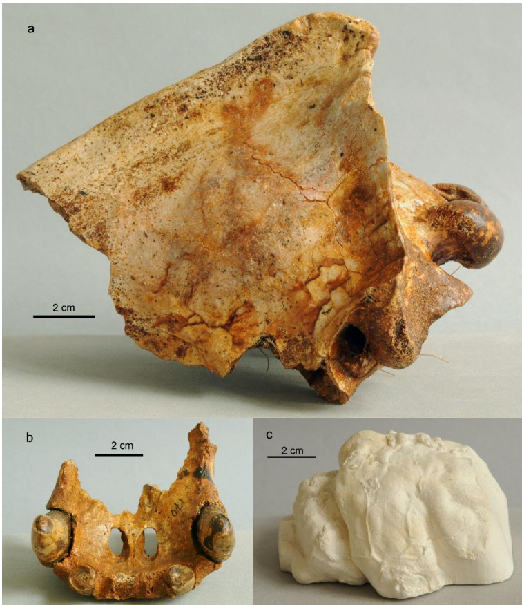
Abbildung 9: Ursus deningeri (MWNH-PLEIS-170a): a) posteriores Schädelfragment ohne Zähne, b) Unterkieferfragment, c) Schädelguss aus Gips von EDINGER (1929).
