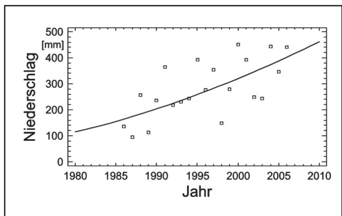
Abb. 3 Jährlicher Niederschlag auf der Farm Kronendaal im S von UG 1 zwischen 1986 und 2006. Über den Erfassungszeitraum hinweg gibt es eine signifikante Zunahme des jährlichen Niederschlages (Y-Quadratwurzel Regressionsmodell, y = (-701,498 + 0,35969 * x)^2 ; Spearman'sche Rangkorrelation, r_s = 0,65 , p < 0,05 ). Quelle: Jannie Burger, Kronendaal.
