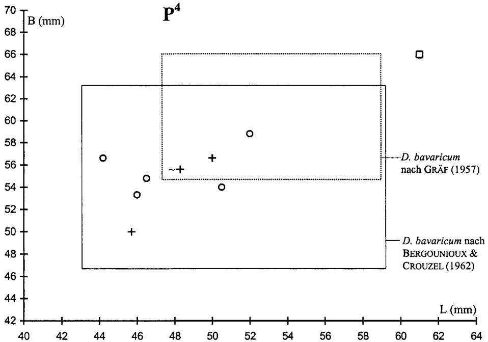
Abb. 5. Deinotherium bavaricum – Längen-Breiten-Diagramm der P 4 der Fundstellen Eggingen-Mittelhart 3 (+, n=3) und Langenau 1 (○, n=5). Zum Vergleich sind die Streubereiche von D. bavaricum nach GRÄF (1957: 154; gestrichelte Linie) und BERGOUNIOUX & CROUZEL (1962: Tab. 5; durchgezogene Linie) sowie ein P 4 aus Benningen bei Memmingen (□, s. DEHM 1949: 19) eingezeichnet.
