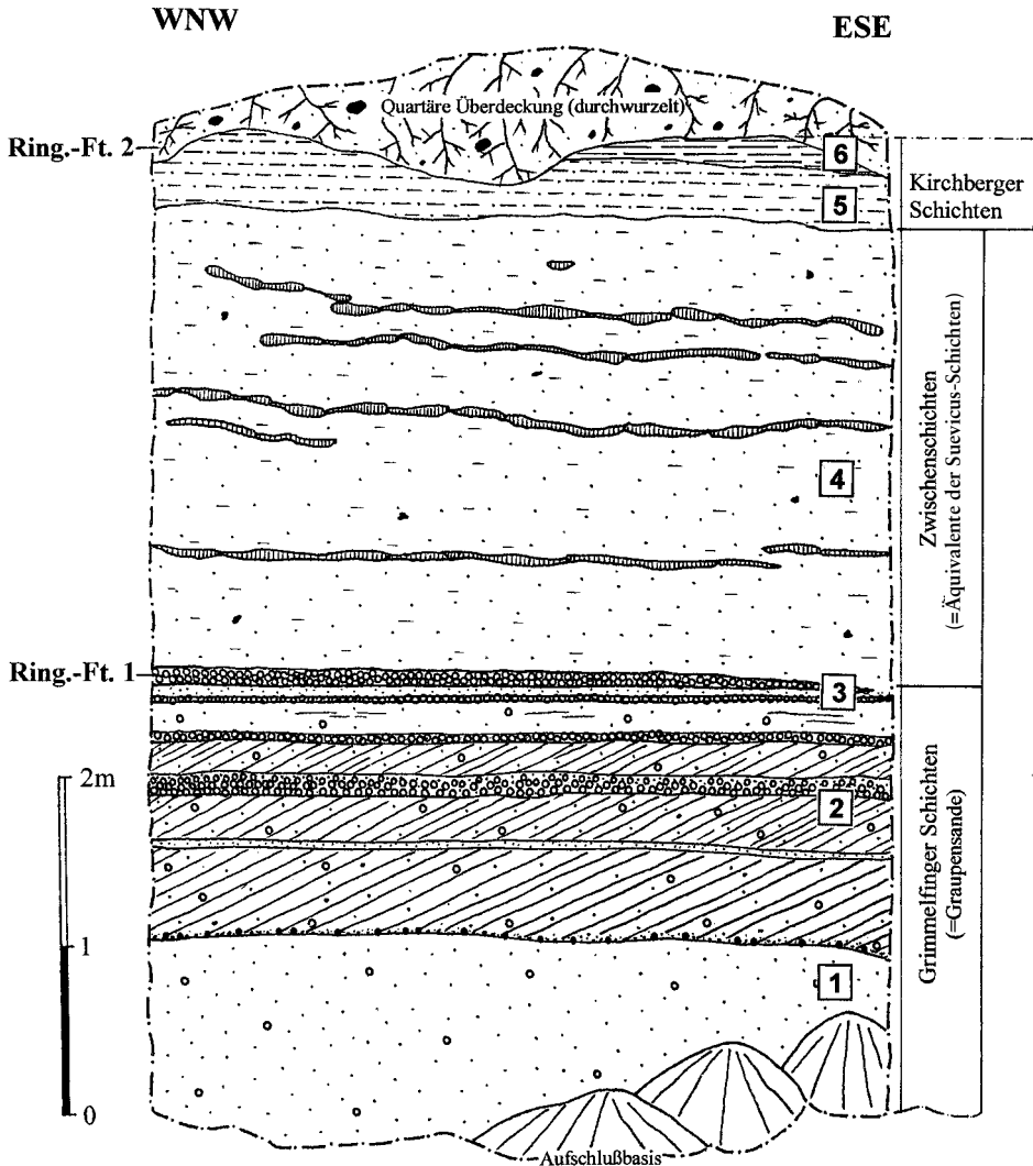
Abb. 3. Skizze des Aufschlusses an der Nordwand der Grube Ringingen-Frontal. Legende: 1 = feinkörnige Graupensande; 2 = schrägeschichtete Graupensande mit Feinkieslagen; 3 = fossilführender Feinkies (Ring.-Ft. 1); 4 = feinsandiger Schluff mit Kalkkonkretionen; 5 = schluffig-feinsandiger Mergel; 6 = Tonmergel (Ring.-Ft. 2).
