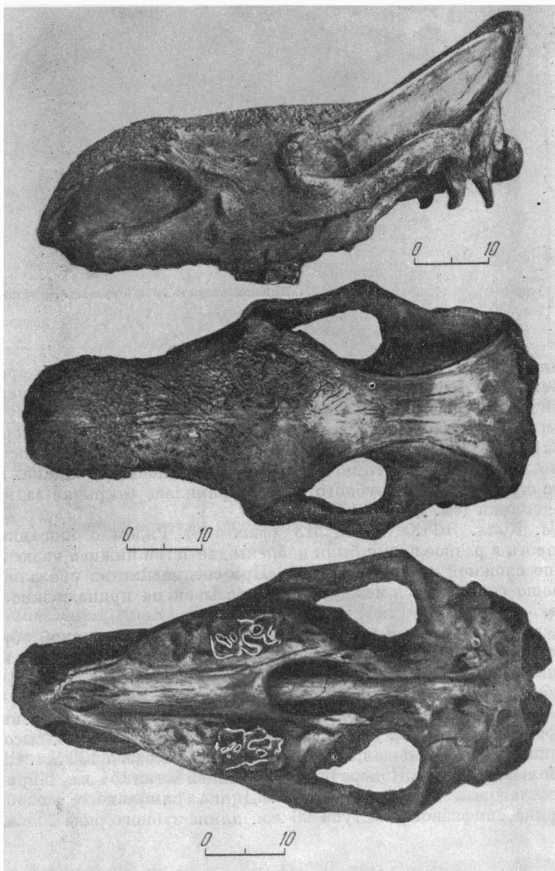
Фиг. 138. Череп № 5 Coelodonta antiquitatis jacuticus Russ. Вид сбоку, сверху и снизу
