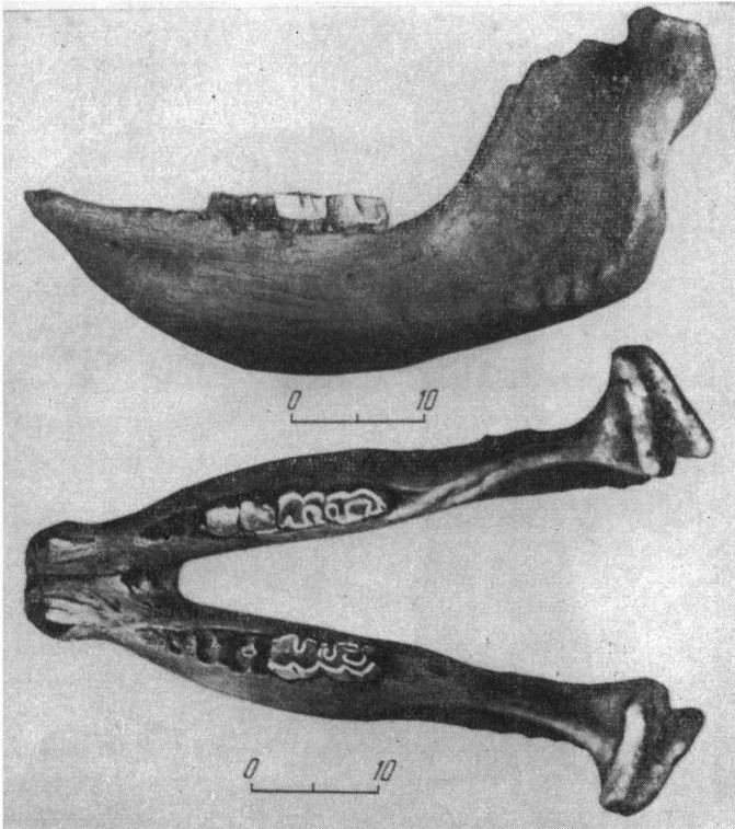
Фиг. 139. Нижняя челюсть № 313 Coelodonta antiquitatis jacuticus Russ. Вид сбоку и сверху
