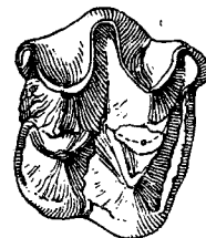
图3 Bothriodon chowi sp. nov. 右 M 3 的冠面视, V. 2599, × 1.
