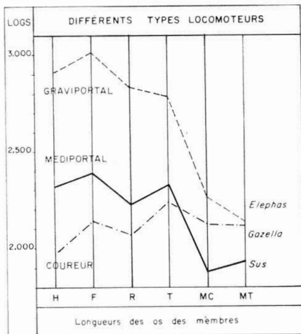
Fig. 1 — Longueurs relatives des os des membres dans les types graviportal (Éléphant), médiportal (Sanglier) et coureur (Gazelle). H = humérus, F = Fémur, R = Radius, T = tibia, MC = troisième métacarpien, MT = troisième métatarsien. Les longueurs sont exprimées en logarithmes décimaux.
