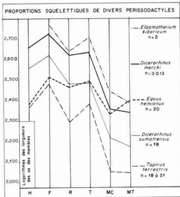
Fig. 2 — Longueurs relatives des os des membres de divers Périssodactyles. Même abréviations que dans la fig. 1 et n = nombre de spécimens.
