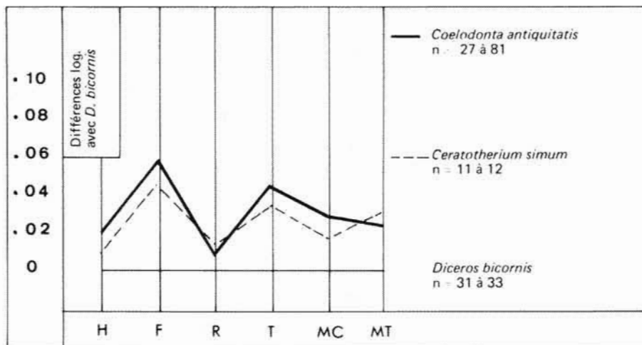
Fig. 4 — Diagramme des rapports des longueurs d'os des membres de divers Rhinocéros. Mêmes abréviations que pour les figures 1 et 2. Ratio-diagrams of Rhinoceroses limb bones lengths. Same abbreviations as in fig. 1 and 2.
